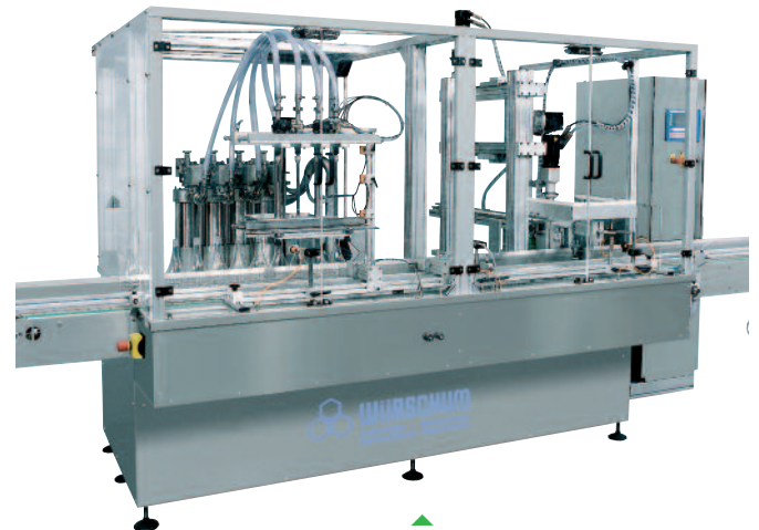
AFS 300-4/AV-200 Abfüll- und Verschließmaschine für flüssige und pastöse Medien.
